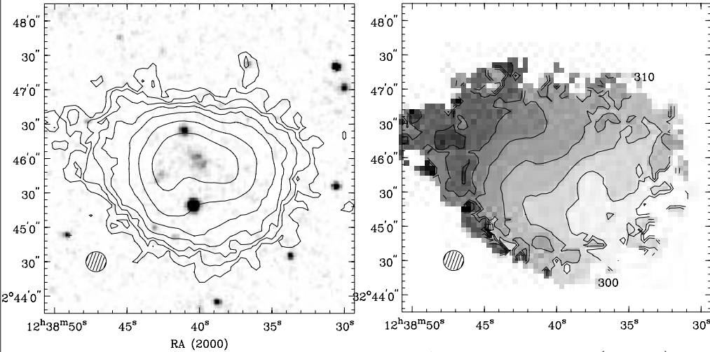
UGCA 292, Young et al. ApJ 592, 111 (2003) M_{\text{HI}} = 10^{7.7} M_{\odot} , M_{\text{HI}}/\mathcal{L}_B \sim 7 M_{\odot}/\mathcal{L}_{\odot}
